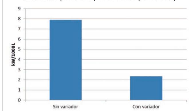
Figura 3. Medición real del consumo eléctrico de la bomba de vacío (ordeño) en una misma granja con el variador de velocidad desconectado (sin variador) o funcionando (con variador)
